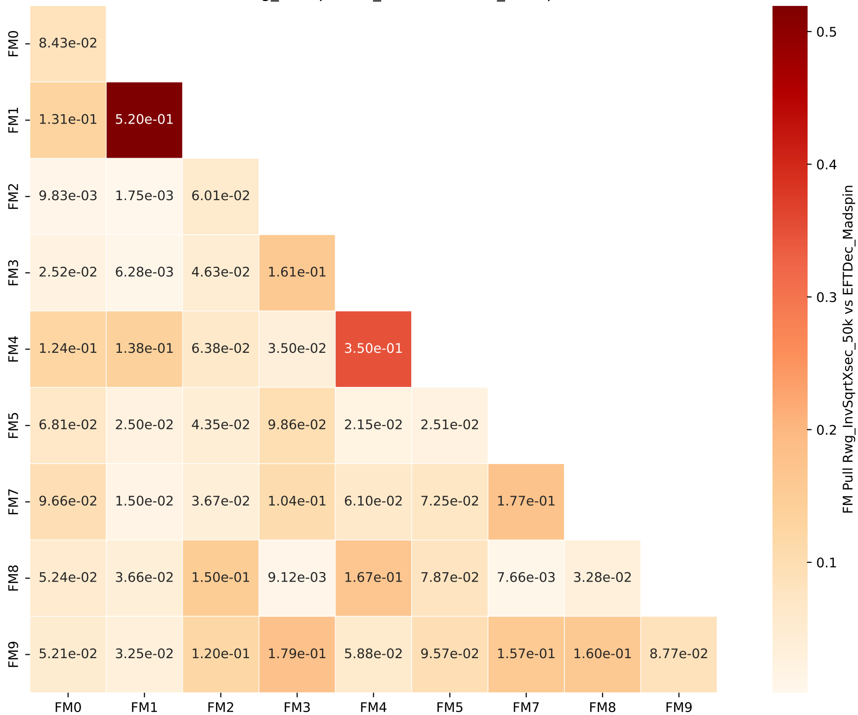
FM Pull Rwg_InvSqrtXsec_50k vs EFTDec_Madspin
